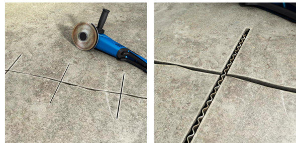
1. Rissflanken aufweiten und alle 15 - 20 cm quer einfräsen. 2. Wellenverbinder einlegen.
