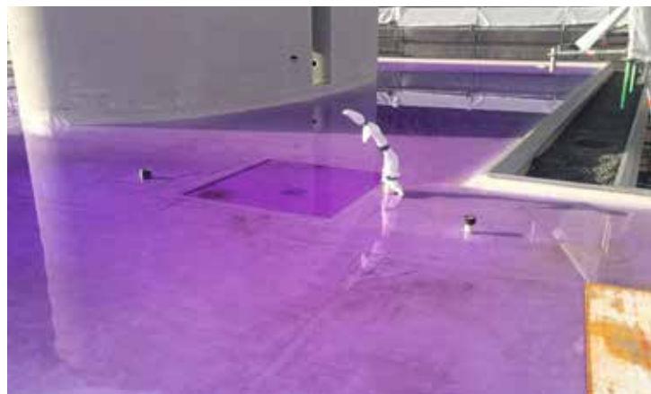
Durch eine Dach-Wässerung konnte die absolute Dichtigkeit geprüft und in einem Abnahmeprotokoll festgehalten werden.
