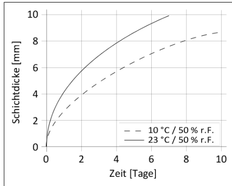
Diagramm 1: Durchhärtegeschwindigkeit Sikaflex®-296
