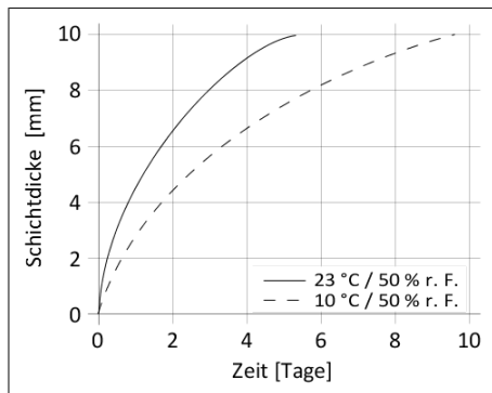
Diagramm 1: Durchhärtengeschwindigkeit Sikaflex®-298 FC
