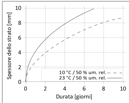
Diagramma 1: velocità di polimerizzazione di SikaTack® PRO
