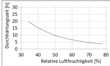
Diagramm 1: Durchhärtszeit für einen 500 µm Klebstofffilm
