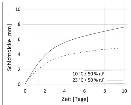
Diagramm 1: Durchhärtengeschwindigkeit Sikaflex®-555
