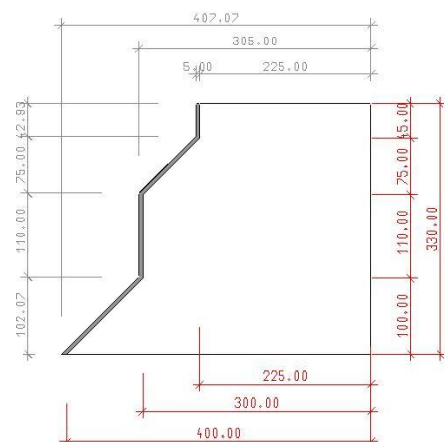
Höhe Konterlatten 86-110 mm
