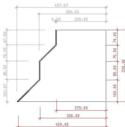
Höhe Konterlatten 60-85 mm
