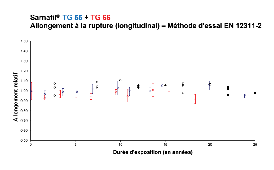
Fig. 9 : Allongement à la rupture (longitudinal) de Sarnafil® TG après exposition sur toit
