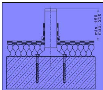
Figura: il sostegno Seculine® Vario fissato con i tasselli
