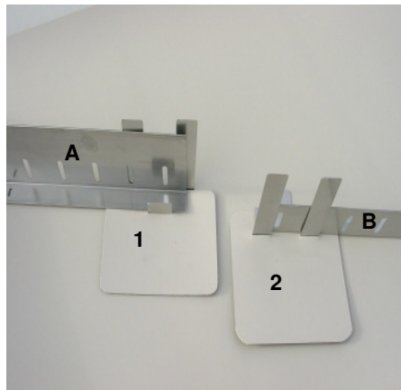
1 Supporto interno 2 Supporto esterno A Profilo paraghiaia 100 mm B Profilo paraghiaia 60 mm
