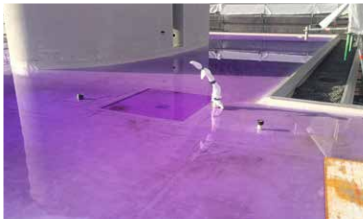
Invaso d'acqua - constatazione dell'assoluta impermeabilità dei tetti - protocollato con piano di controllo
