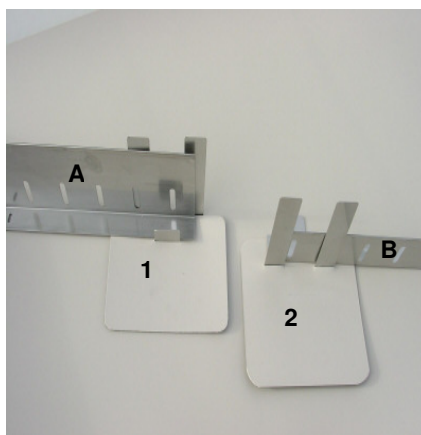
1 Support de montage intérieur 2 Support de montage extérieur A Cornière à gravier 100 mm B Cornière à gravier 60 mm
