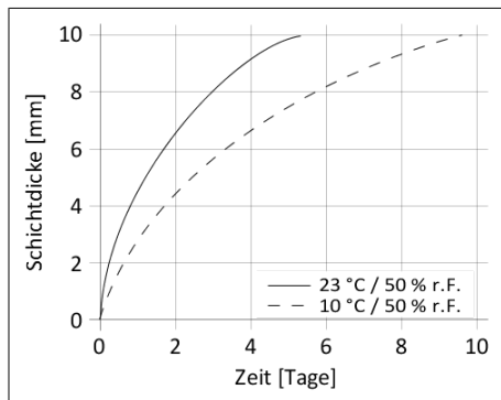
Diagramm 1: Durchhärtengeschwindigkeit Sikaflex®-228
