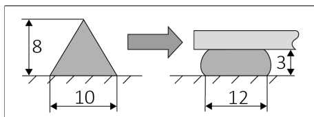
Abbildung 1: Empfohlener Klebstoffauftrag
