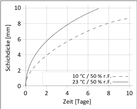
Diagramma 1: velocità di polimerizzazione di Sikaflex®-621
