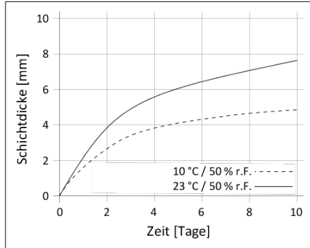
Diagramm 1: Durchhärtgeschwindigkeit Sikaflex®-529 Evolution
