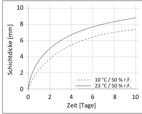
Diagramm 1: Durchhärtageschwindigkeit von Sikaflex®-292i
