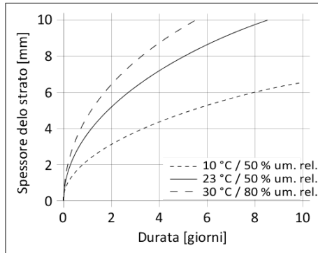
Diagramma 1: velocità di polimerizzazione di Sikaflex®-254
