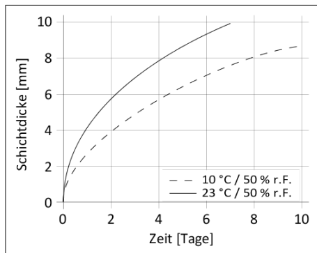
Diagramm 1: Durchhärtungsgeschwindigkeit Sikaflex®-295 UV
