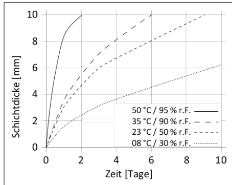
Diagramm 1: Durchhärtegeschwindigkeit Sikasil® AS-70
