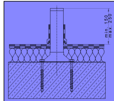
Abb. Aufgedübelte Seculine®Vario-Stütze
