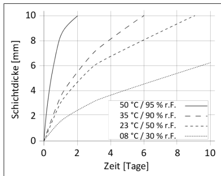
Diagramm 1: Aushärtengeschwindigkeit Sikasil® SG-20
